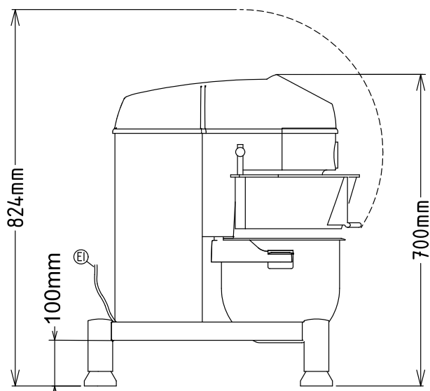
Côté
